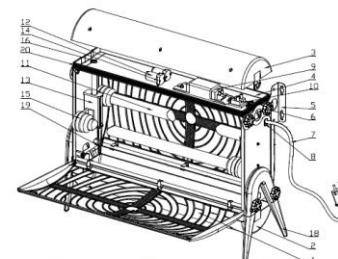
Rys. 1 Pułapka świetlna na owady DEAL-004 eco
